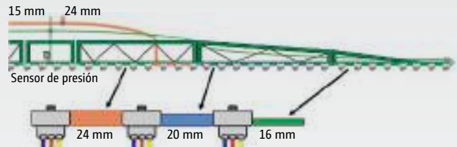
Circulación de alta presión SCF pro con línea de pulverización cónica en el ejemplo de AmaSwitch
