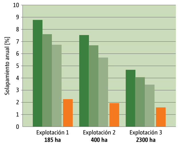
Equipación de las máquinas de aplicación de fitosanitarios: ■ 9 anchos parciales ■ 11 anchos parciales ■ 13 anchos parciales ■ Control de boquillas individuales con anchos parciales de 50 cm
