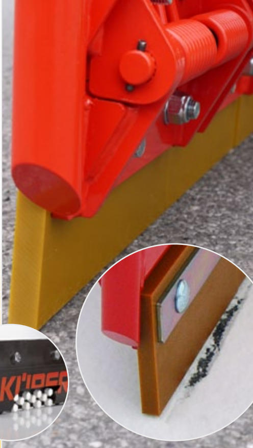
Необледеневающие пружинящие щитки, серийно с кромочными отражателями (в ассортименте различные изнашивающиеся планки)
