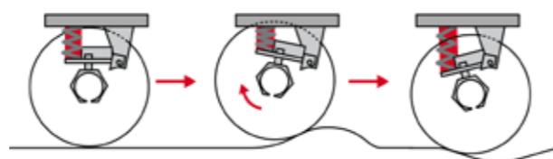
Die Achsfederung gleicht Bodenunebenheiten optimal aus.
