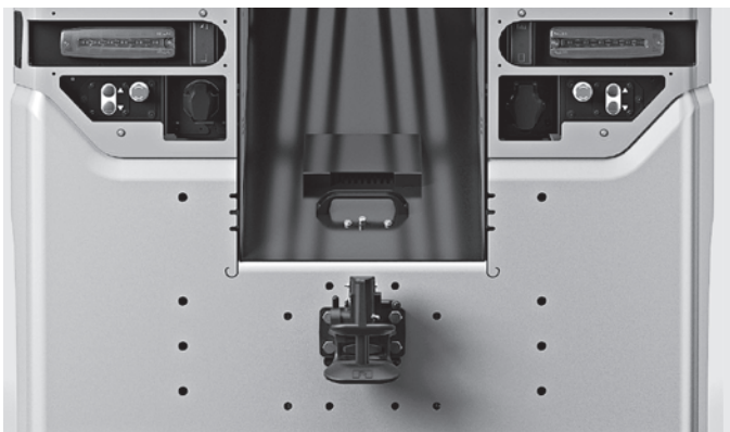
Für sicheres und effizientes An- und Abkuppeln sorgen Rückasteinrichtungen am Heck
