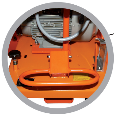
Schnitttiefeinstellung über Fußpedal
