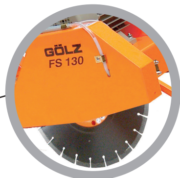
Sägeblattdurchmesser bis zu 400 mm (Schnitttiefe von 145 mm)
