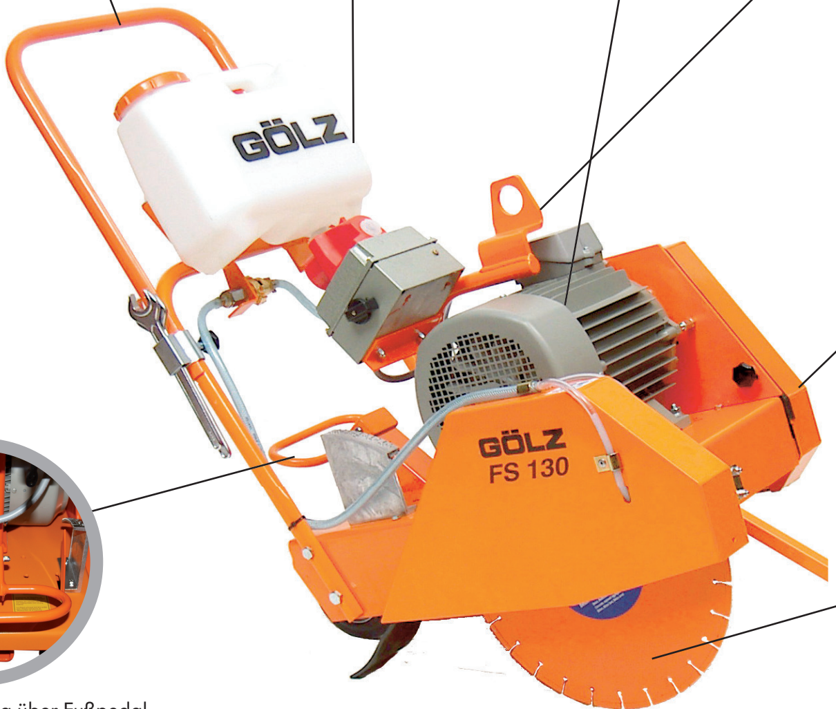
Schnitttiefeinstellung über Fußpedal
