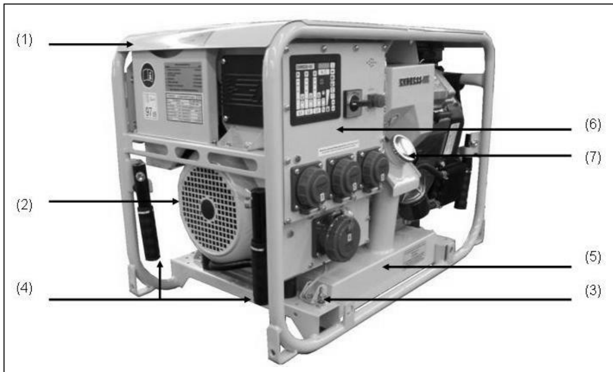
Abb. 3-2: Bestandteile der Bedien- und Generatorseite
