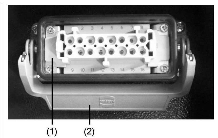
Abb. 5-4: Fernstarteinrichtung mit Harting-Stecker
