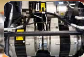
Moteurs de pompe et traction de type fermé indice de protection IP43 simple et puissant
