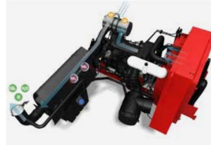
● Oxidation ● Reaktion
