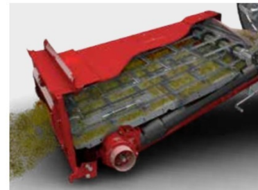
Der leistungsstarke Schrägförderer verarbeitet selbst die dichten Materialströme der größten Schneidwerke ohne Probleme
