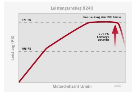
Leistungsanstieg (8240)
