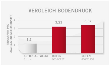
Case IH Raupenlaufwerke bewähren sich seit Jahren auf Quadtrac Schleppern.
