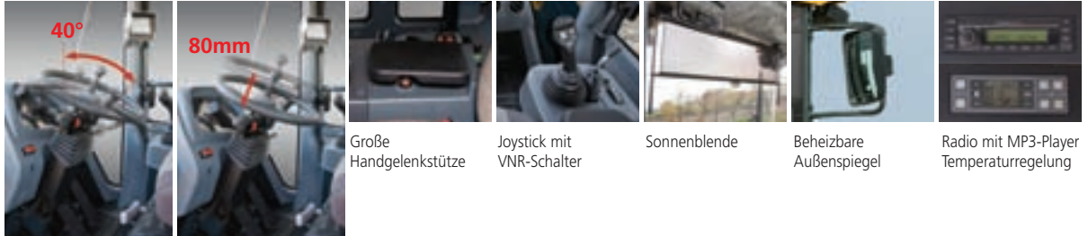
Neigbare Teleskop-Lenksäule
