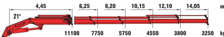
a5 14,21 m max. hydraulische Reichweite ( Arm gestreckt / max. outreach (horizontal position)
