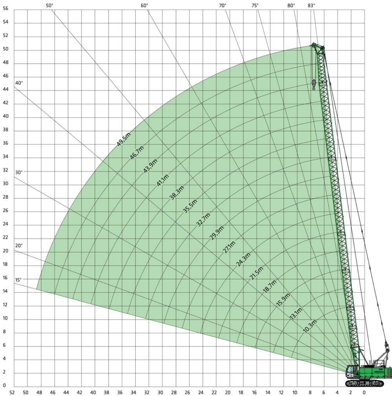
Auslegerkonfiguration
