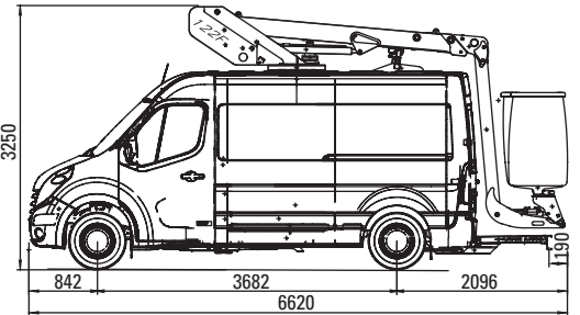
122F sur porteur RENAULT MASTER
